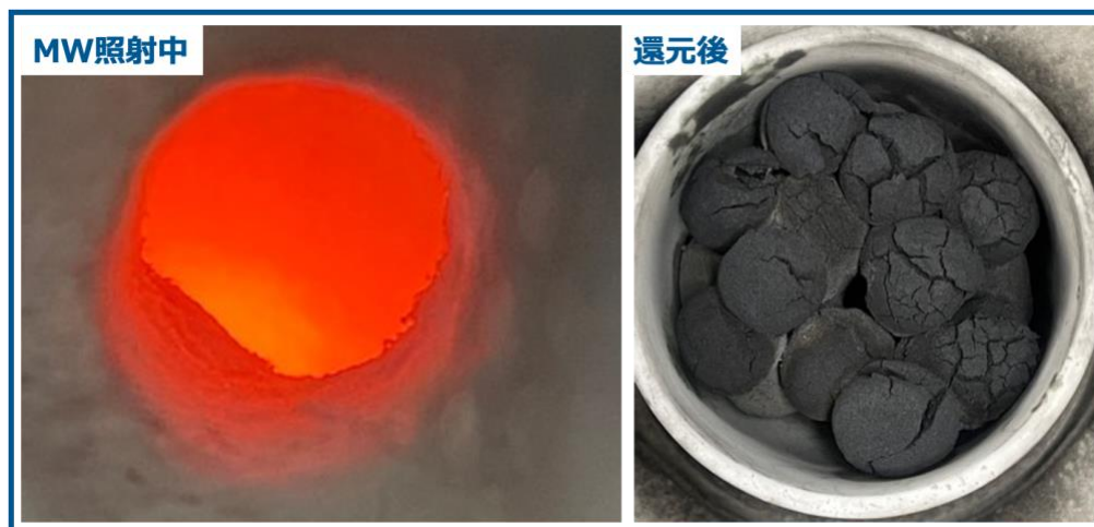
ラボでのマイクロ波による鉄鉱石の還元
